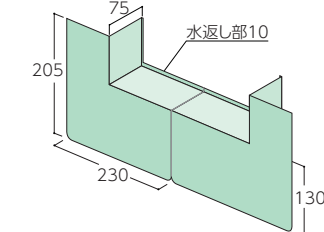
角部材75
