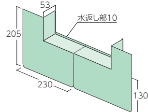
角部材53
